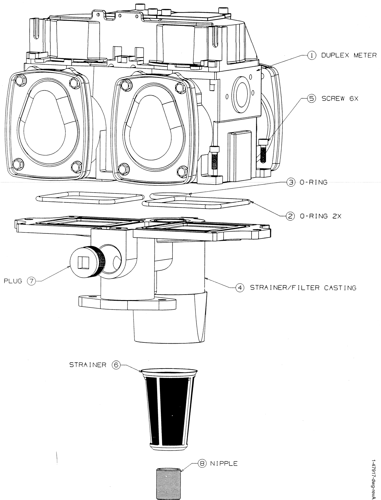
FIGURE 24. 1-47917-DWG - IMETER MODULE
